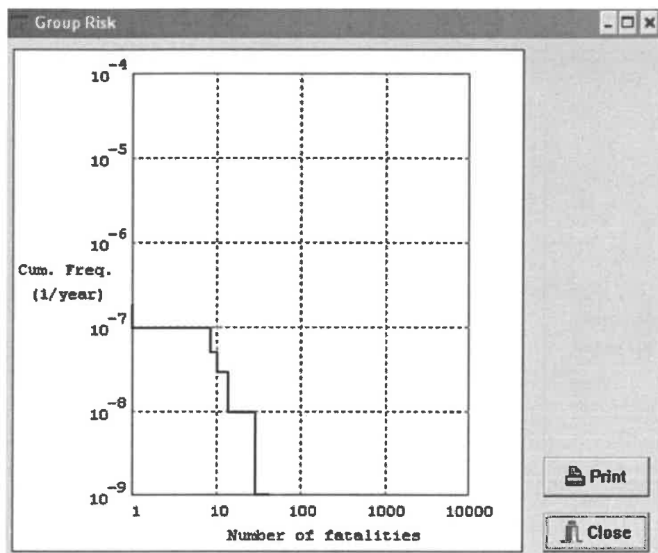
A szcenáriók F-N görbéje (állandó külsős munkavállalók figyelmen kívül hagyásával)
