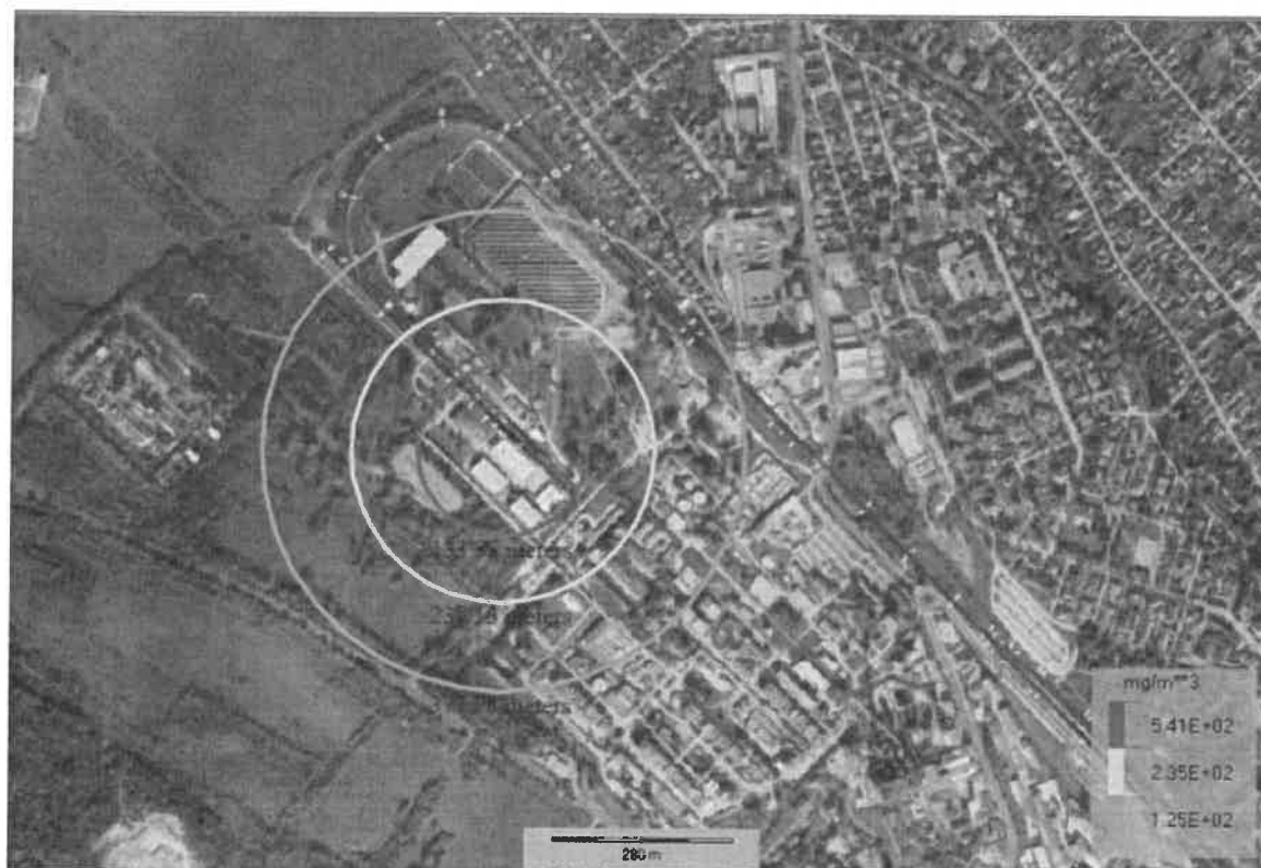
Nitrogén-oxid kikerüléséhez tartozó izokoncentrációs görbék
