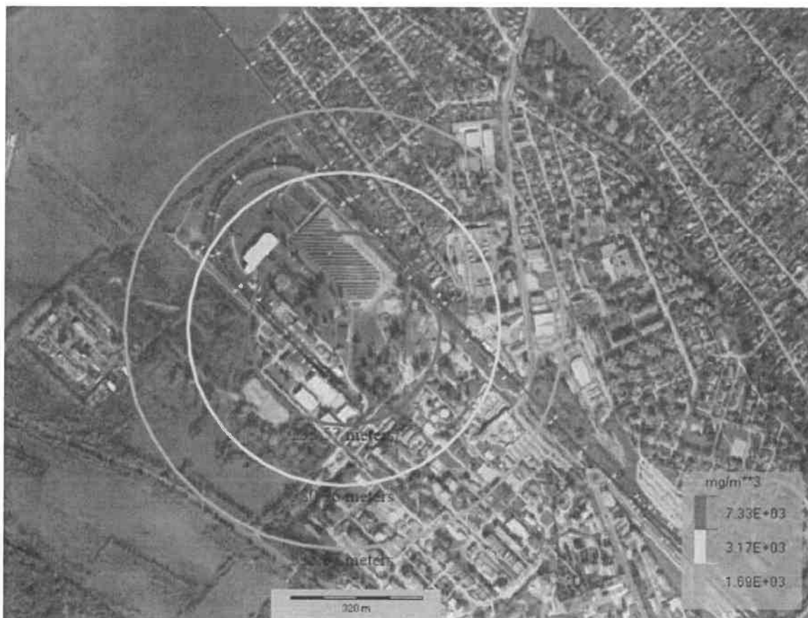
Sósavgáz kikerülésének izokoncentrációs görbéi
